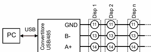
Comunicazione su RS485
