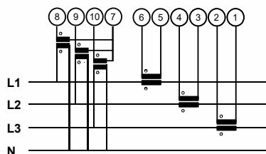
Trifase, 4 fili, connessione con 3 TA e 3 TV
