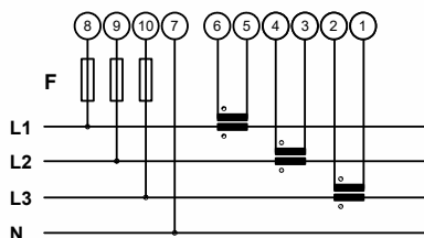
Trifase, 4 fili, connessione con 3 TA
