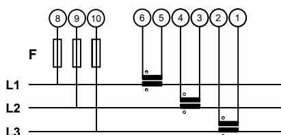
Trifase, 3 fili, connessione con 3 TA
