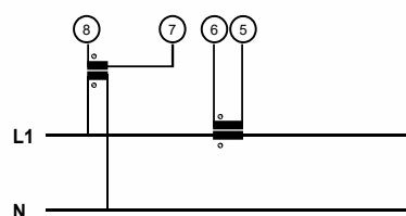
Monofase, 2 fili, connessione con 1 TA e 1 TV
