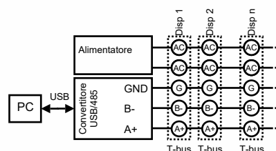
Comunicazione RS485 su connettore T-Bus
