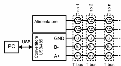
Alimentazione e comunicazione RS485 su connettore T-Bus
