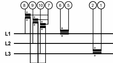
Trifase, 3 fili, connessione con 2 TA e 3 TV (Aron)
