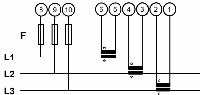
Trifase, 3 fili, connessione con 3 TA
