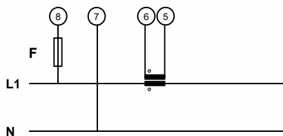
Monofase, 2 fili, connessione con 1 TA
