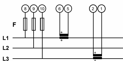
Trifase, 3 fili, connessione con 2 TA (Aron)
