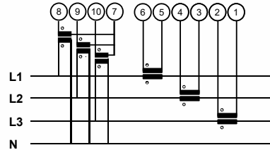
Trifase, 4 fili, connessione con 3 TA e 3 TV
