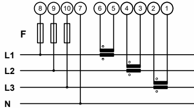
Trifase, 4 fili, connessione con 3 TA
