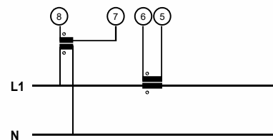
Monofase, 2 fili, connessione con 1 TA e 1 TV
