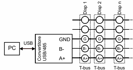
Comunicazione RS485 su connettore T-Bus (richiede l'accessorio opzionale)
