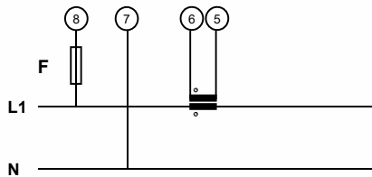
Monofase, 2 fili, connessione con 1 TA
